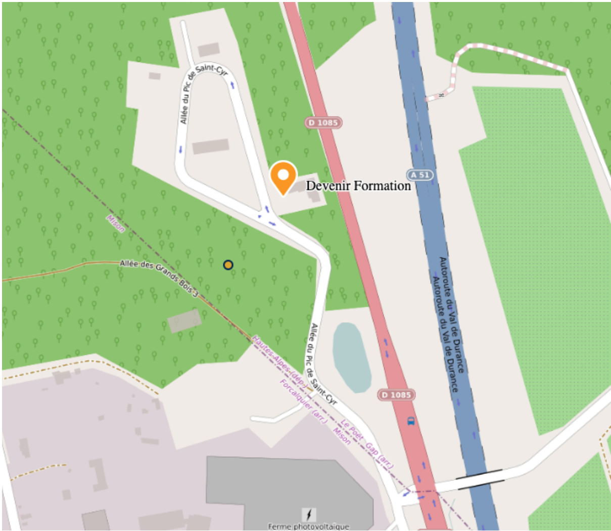
Géoportail carte "OpenStreetMap monde" (02/09/2025)
